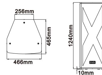
PR52全频音箱
