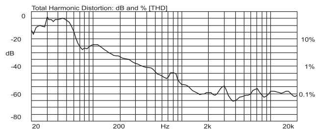
总谐波失真曲线：
