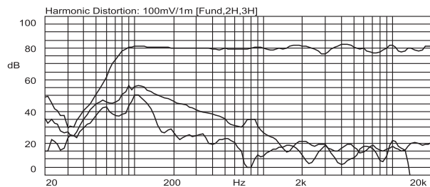
频响曲线，二次谐波和三次谐波失真曲线：
