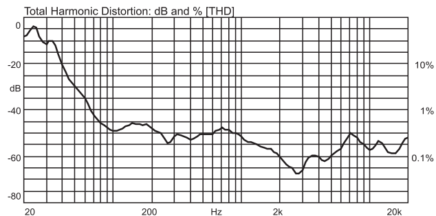
☑ 总谐波失真曲线：
