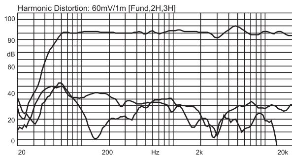
☑ 频响曲线，二次谐波和三次谐波失真曲线：
