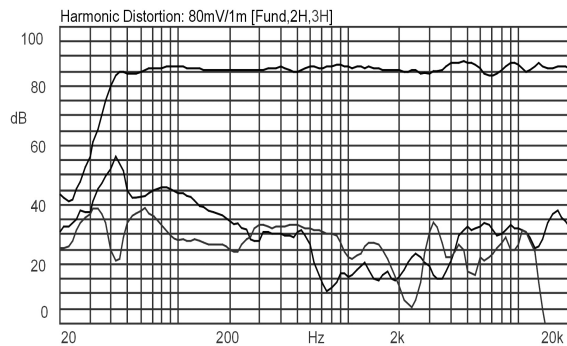
频响曲线，二次谐波和三次谐波失真曲线：
